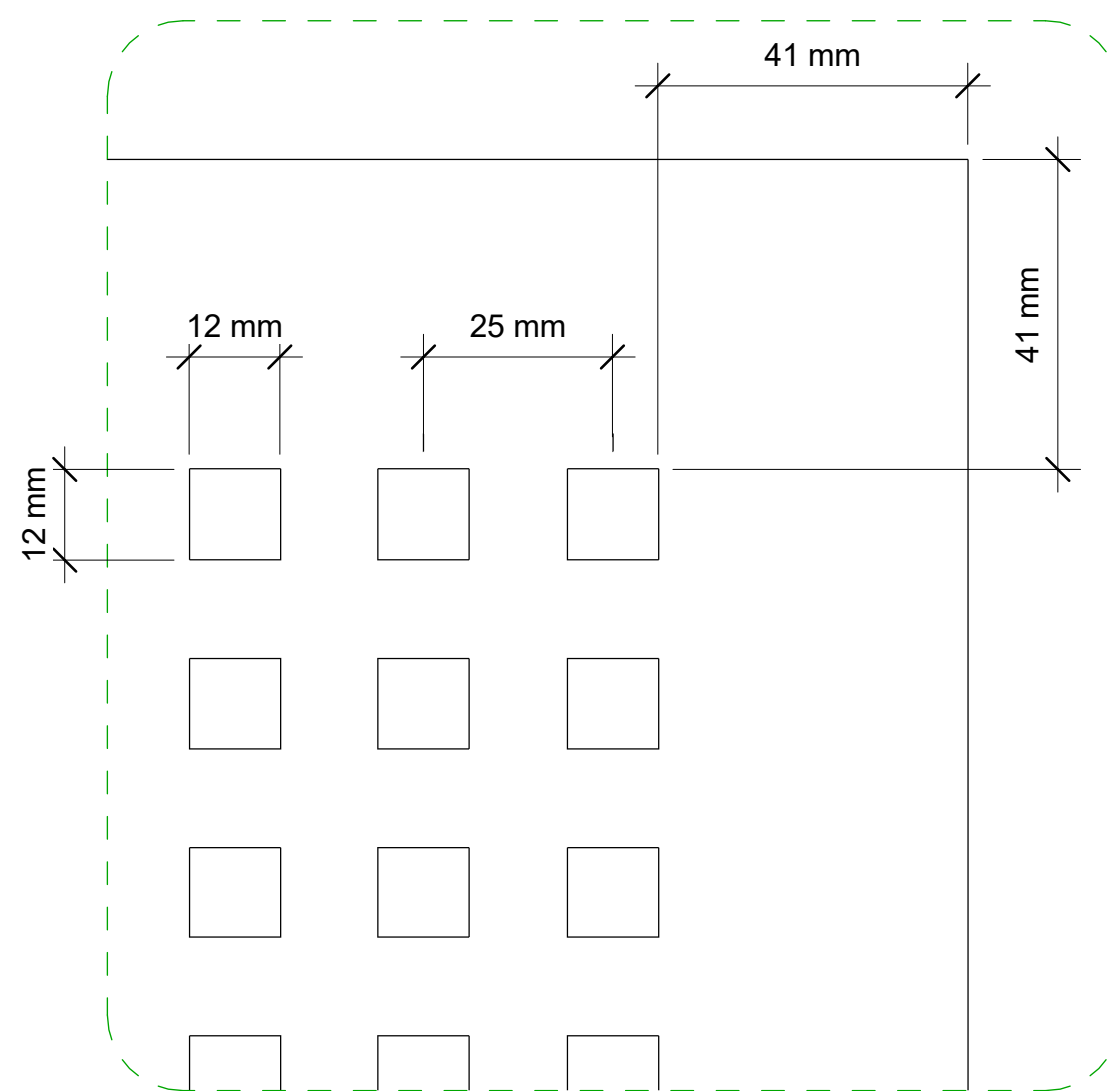
3 Detail 1 1 : 1
